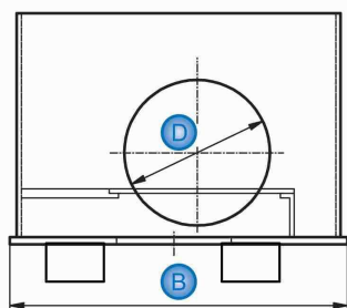
Seitenansicht links (Ablauf Kanal)
